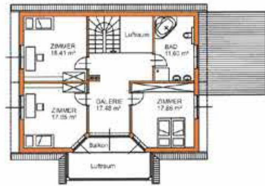
Grundriss Obergeschoss
