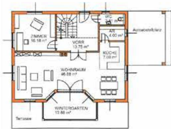
Grundriss Erdgeschoss
